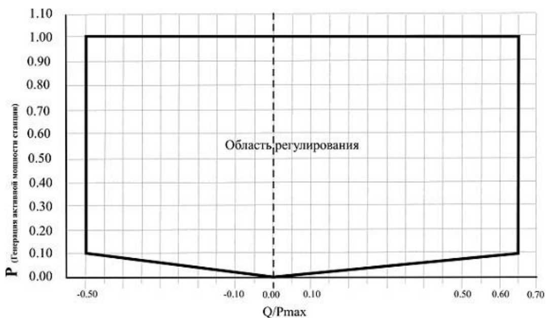
Рисунок 5 Зависимость регулировочного диапазона по реактивной мощности СЭС от ее фактической генерации
