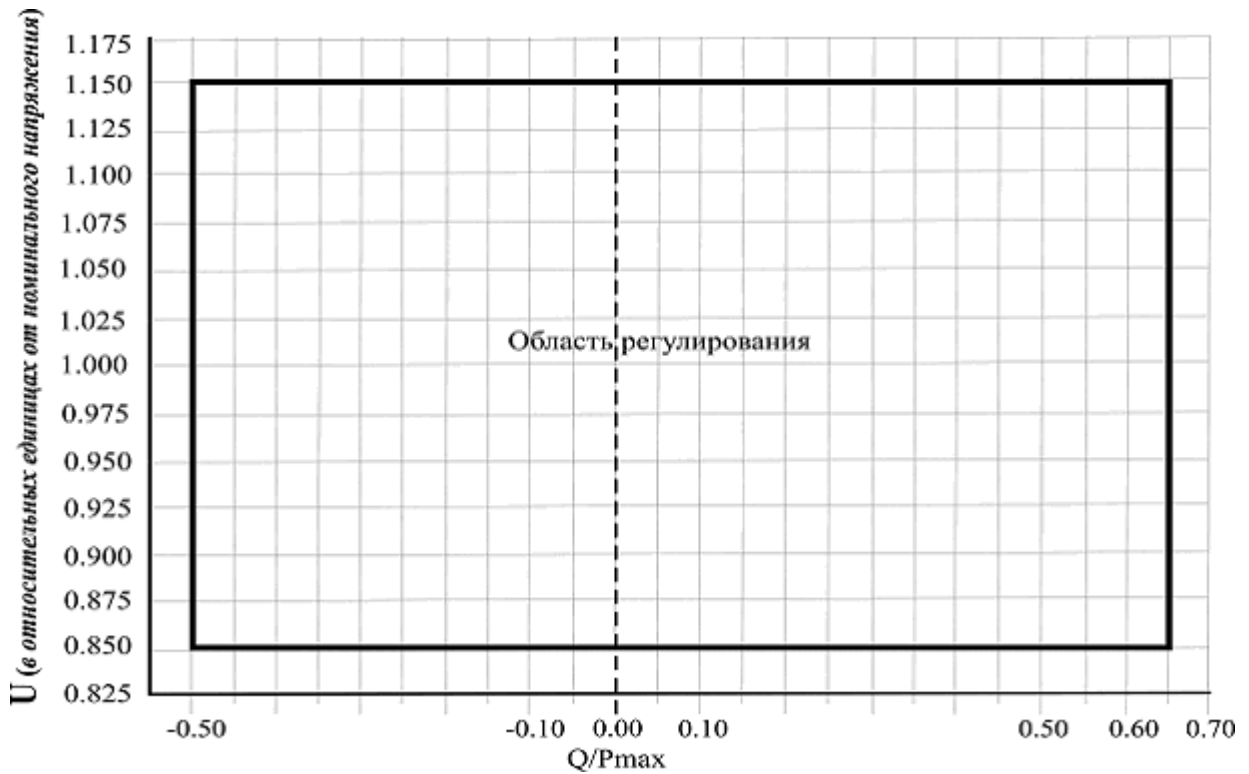
Рисунок 3. Зависимость регулировочного диапазона по реактивной мощности СЭС от фактического напряжения в точке подключения.
